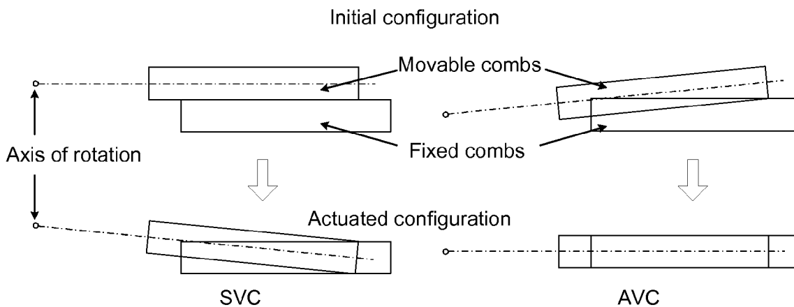
FIG. 23A
