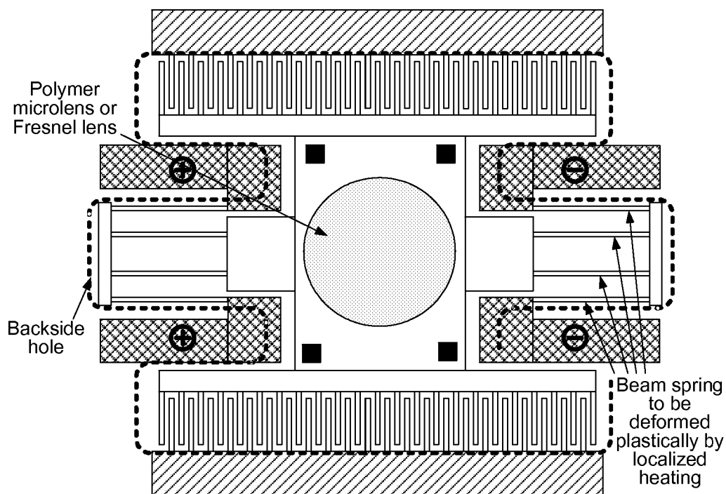
FIG. 21A
