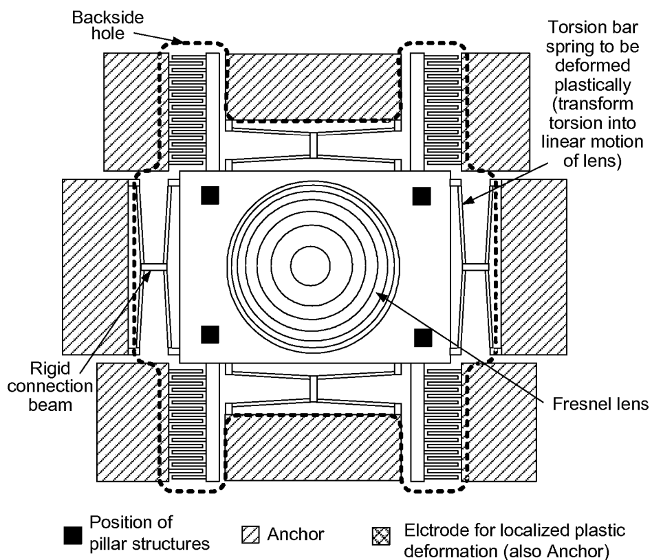
FIG. 21B
